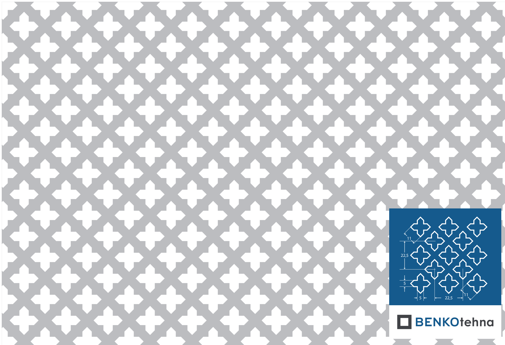
CL - Križna 11×22,5: odprtost = 41,23%
