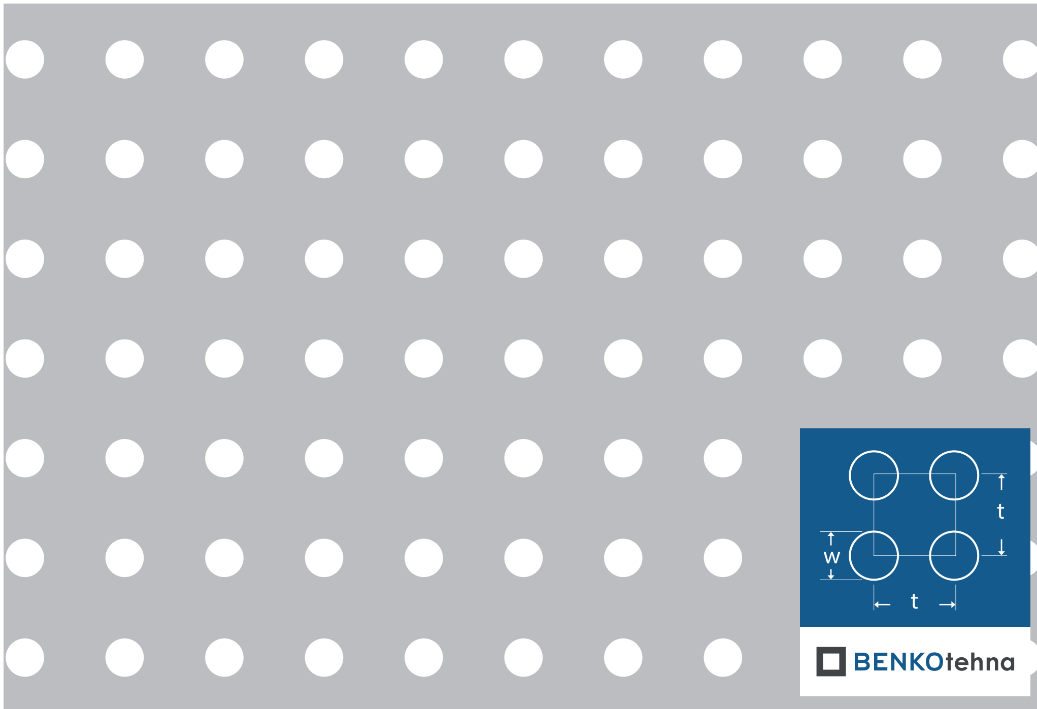
Okrogla vrstna Ov 10-25,98: w = 10,0 \text{ mm} | t = 25,98 \text{ mm} | odprtost = 11,63%
