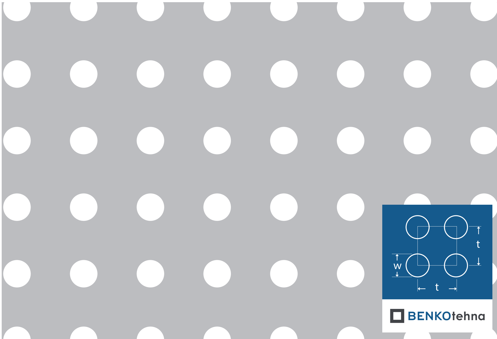
Okrogla vrstna Ov 15-36,38: w = 15,0 mm | t = 36,38 mm | odprtost = 13,35%
