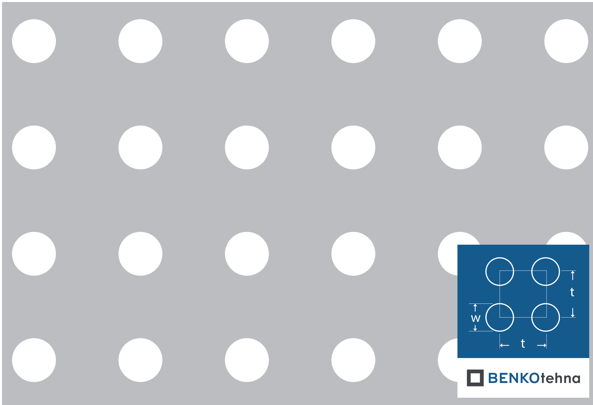
Okrogla vrstna Ov 20-48,5: w = 20,0 \text{ mm} | t = 48,5 \text{ mm} | odprtost = 13,35%
