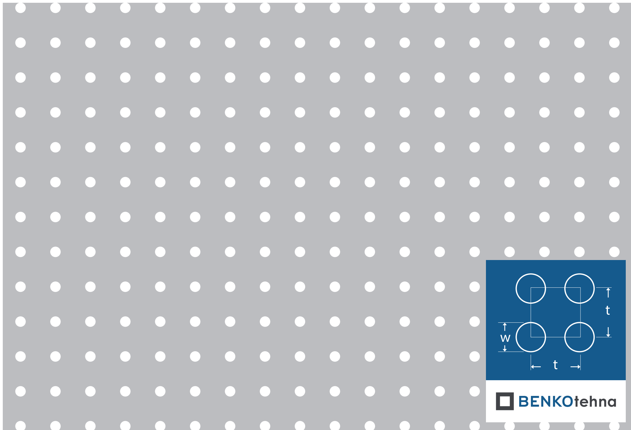
Okrogla vrstna Ov 4,5-15: w = 4,5 \text{ mm} | t = 15,0 \text{ mm} | odprtost = 7,07%
