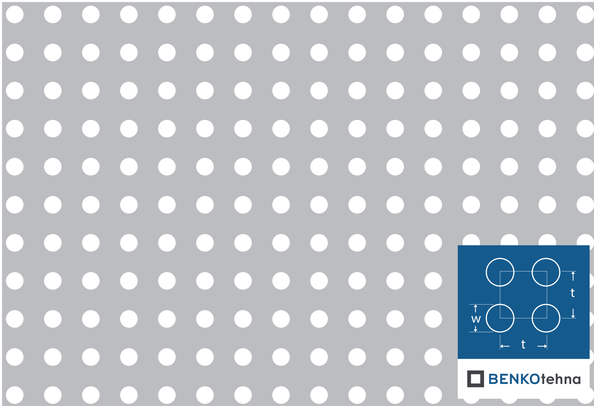
Okrogla vrstna Ov 8-17,32: w = 8,0 \text{ mm} | t = 17,32 \text{ mm} | odprtost = 16,75%
