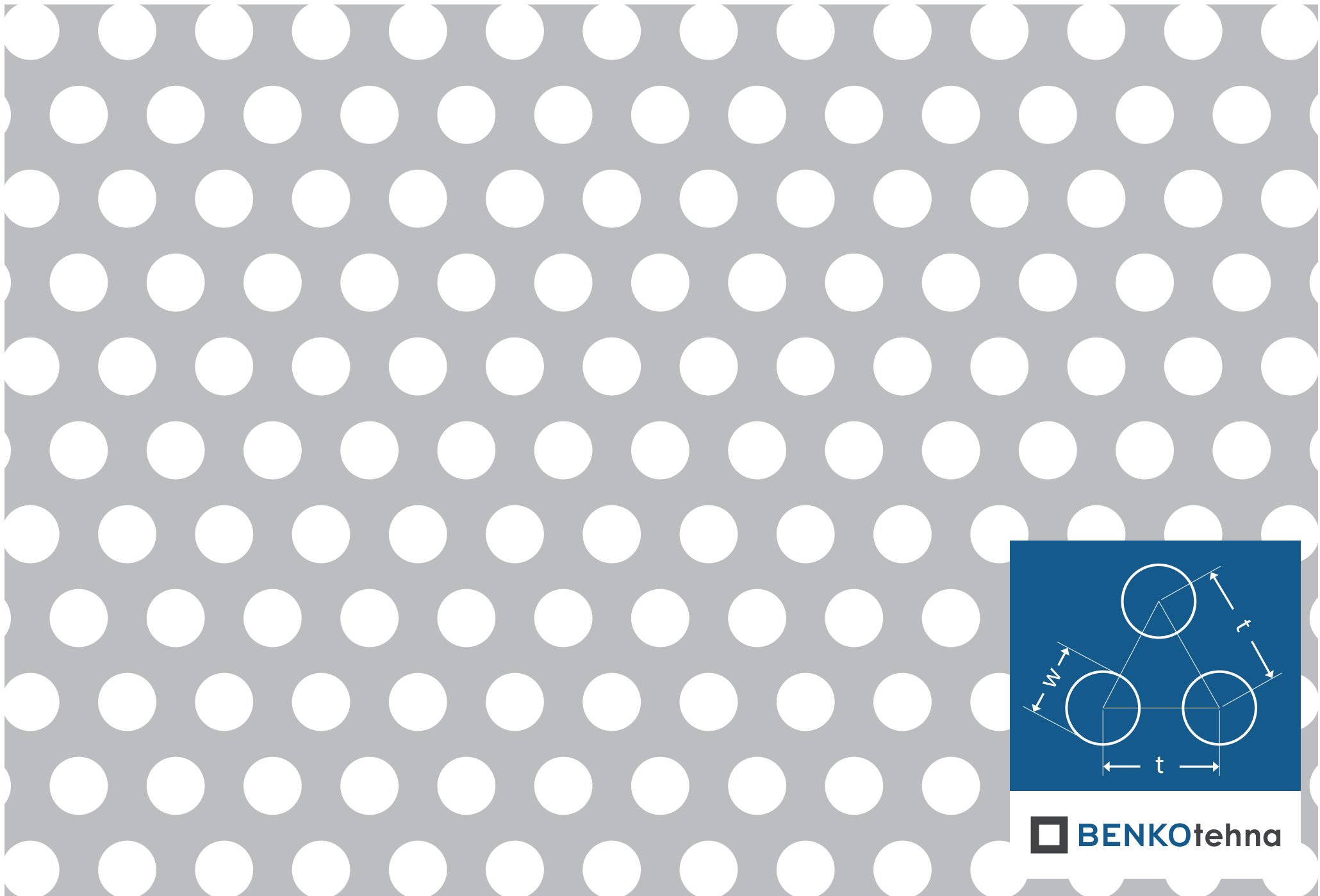
Okrogla zamaknjena Oz 12-20: w = 12,0 \text{ mm} | t = 20,0 \text{ mm} | odprtost = 32,65%
