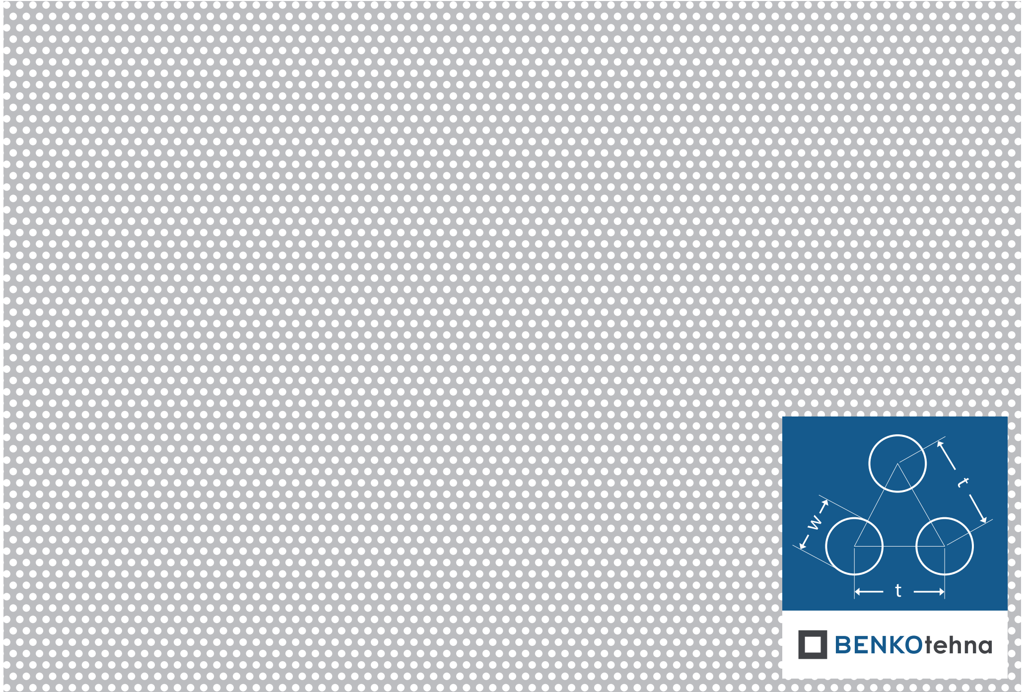
Okrogla zamaknjena Oz 2-3,5: w = 2,0 \text{ mm} | t = 3,5 \text{ mm} | odprtost = 29,62%
